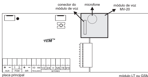
figura 11: instalação do módulo de voz
