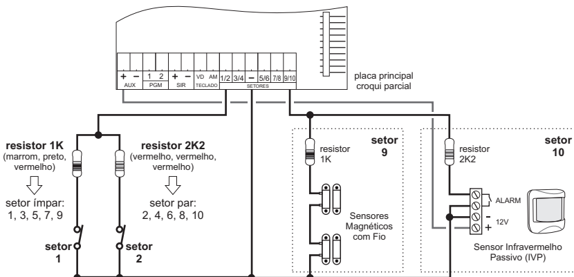
figura 8: ligação de sensores com fio
