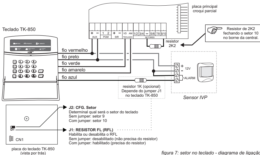
figura 7: setor no teclado - diagrama de ligação
