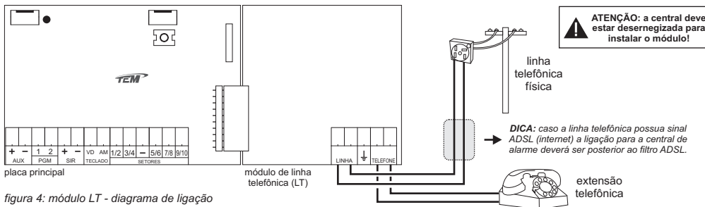
figura 4: módulo LT - diagrama de ligação
