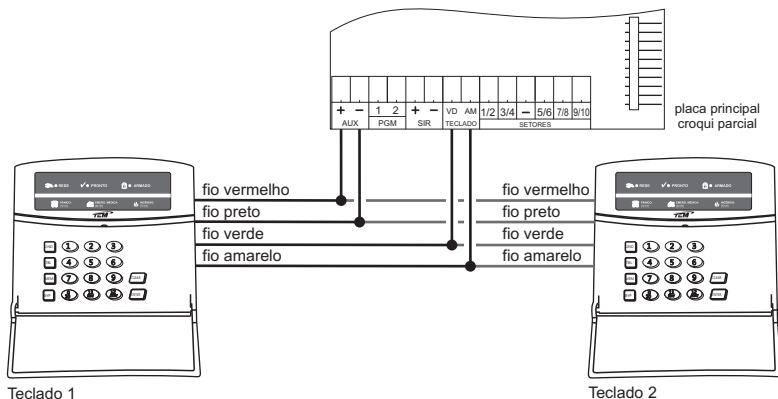
figura 6: teclado externo - diagrama de ligação
