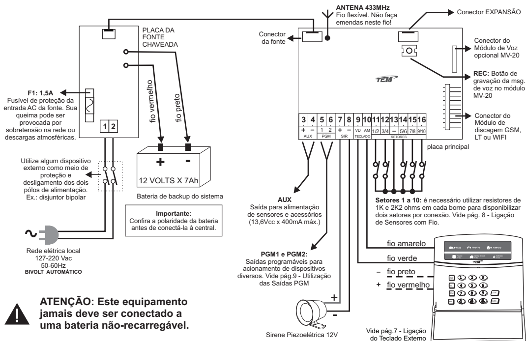
figura 3: diagrama de fiação
