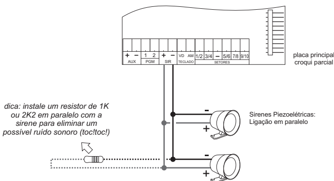
figura 9: ligação de sirenes
